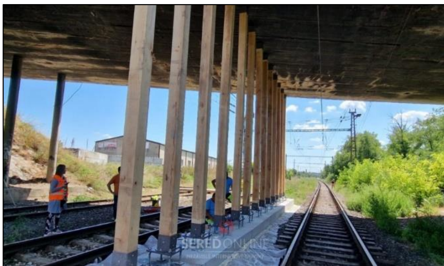
Havarijný stav mosta v Sereďi
